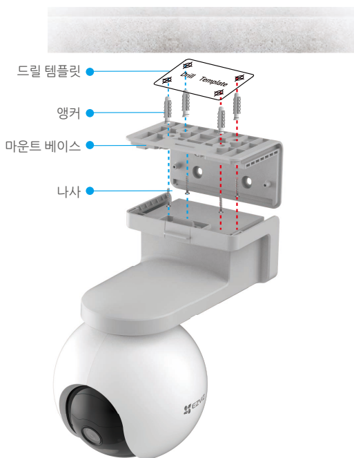
그림 1 천장 장착
