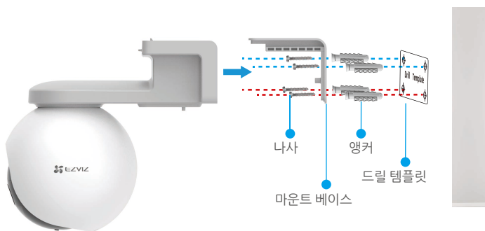
그림 2 벽 장착
